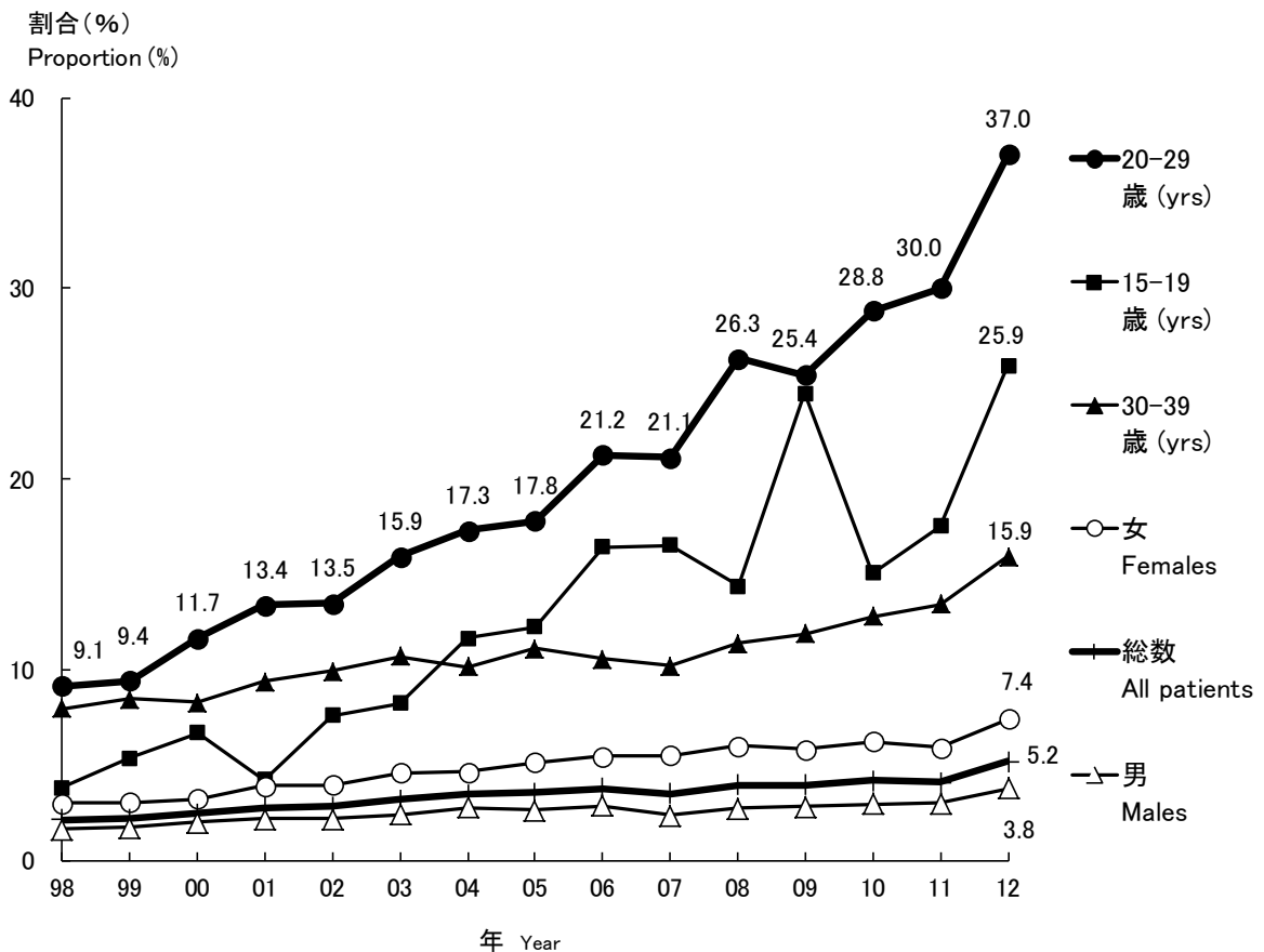
図3 新登録結核患者に占める外国生まれ結核患者割合の推移、性別・特定年齢階層別、1998～2012年 Fig. 3 Annual trend of proportion of foreign-borns among newly notified tuberculosis patients, by age group, from 1998 to 2012
