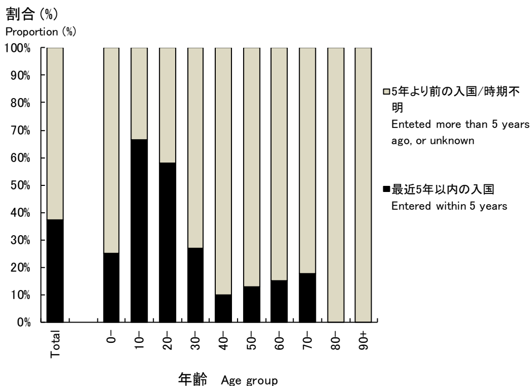
図 4 外国生まれ結核患者の入国時期別割合、年齢階層別、2012年 Fig. 4 Proportion of foreign-born tuberculosis patients, by age group and time of entry to Japan, in 2012
