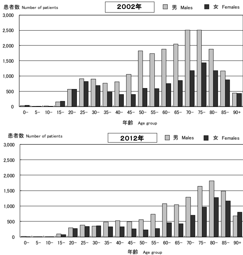
図 2 新登録結核患者数の年齢分布, 性別, 2002年・2012年 Fig. 2 Age distribution of newly notified tuberculosis patients by sex in Japan, in 2002 and in 2012
